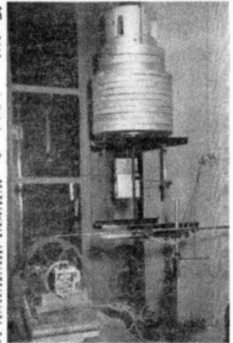
En la fotografía, uno de los sismógrafos instalados en el Observatorio de Gijón. De los que sirven para registrar los movimientos de la corteza terrestre. Son los más sensibles instalados para registrar en la zona del puerto de Gijón.
