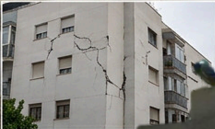
GRIETAS ESTRUCTURALES
